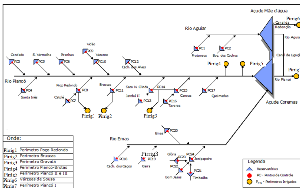
Figura 2 - Sistema de reservatórios com suas demandas e pontos de controle para outorga na Bacia do Rio Piancó
