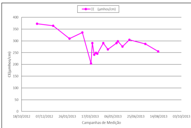
Figura 7 – Variação da condutividade elétrica (CE) nas águas do Rio Piranhas em Pombal-PB. Fonte: autor, 2013.
