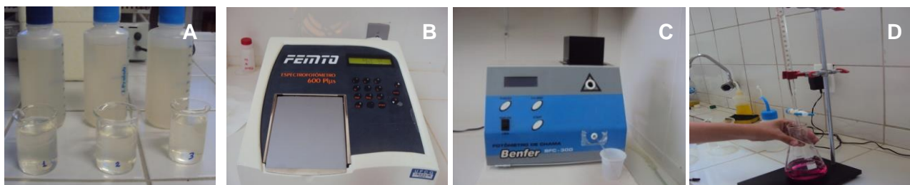
Figura 3 – (A): Amostras de água coletadas, (B): Determinação de Nitrogênio Total e Fósforo Total, (C): Determinação de sódio e potássio e (D): Determinação de cálcio e magnésio. Fonte: Autor, 2013.
