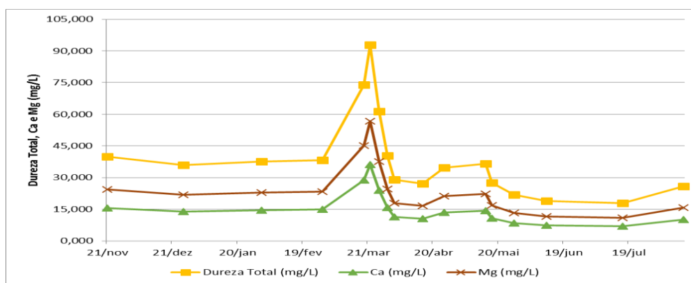
Figura 4 – Variação das concentrações de Dureza Total (mg/L), Ca (mg/L) e Mg (mg/L) no período estudado. Fonte: Autor, 2013.
