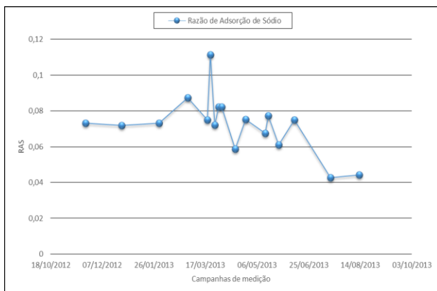
Figura 6 – Variação da RAS nas águas do Rio Piranhas em Pombal-PB. Fonte: autor, 2013.
