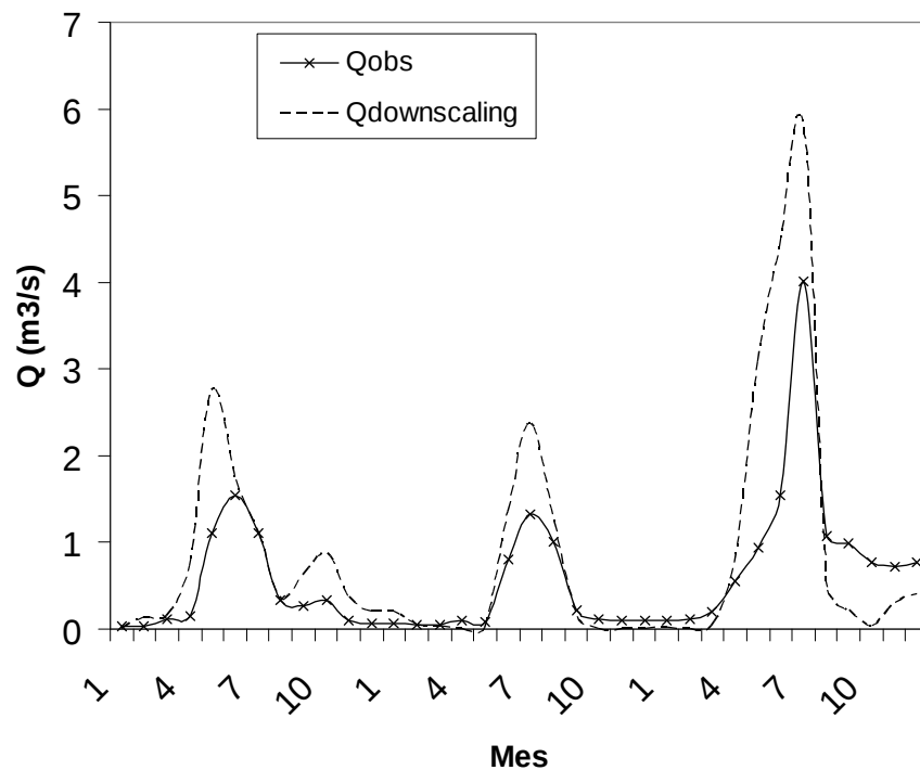
Figura 8 – Hidrograma observado e simulado para o posto Faz Pão de Açúcar utilizando os parâmetros calibrados na Fazenda Cajueiro – 1986-1988 – NS = -0,10; PBIAS = 41,68%
