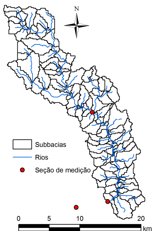
Figura 3 – Discretização em 112 sub-bacias seção Fazenda Cajueiro
