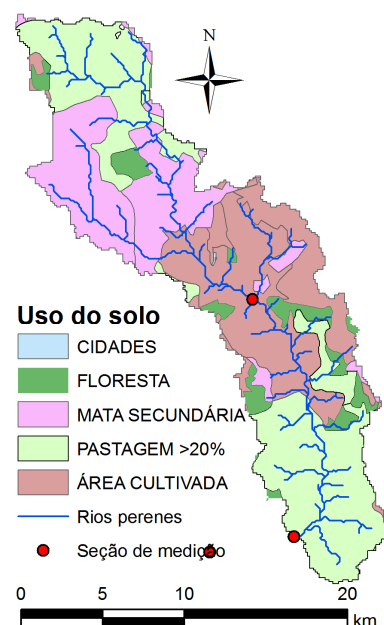
Figura 2 - Uso do solo na sub-bacia do Rio Japarutuba-Mirim
