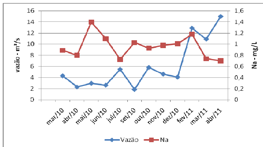
Figura 8 – Relação entre concentração de sódio e a vazão
