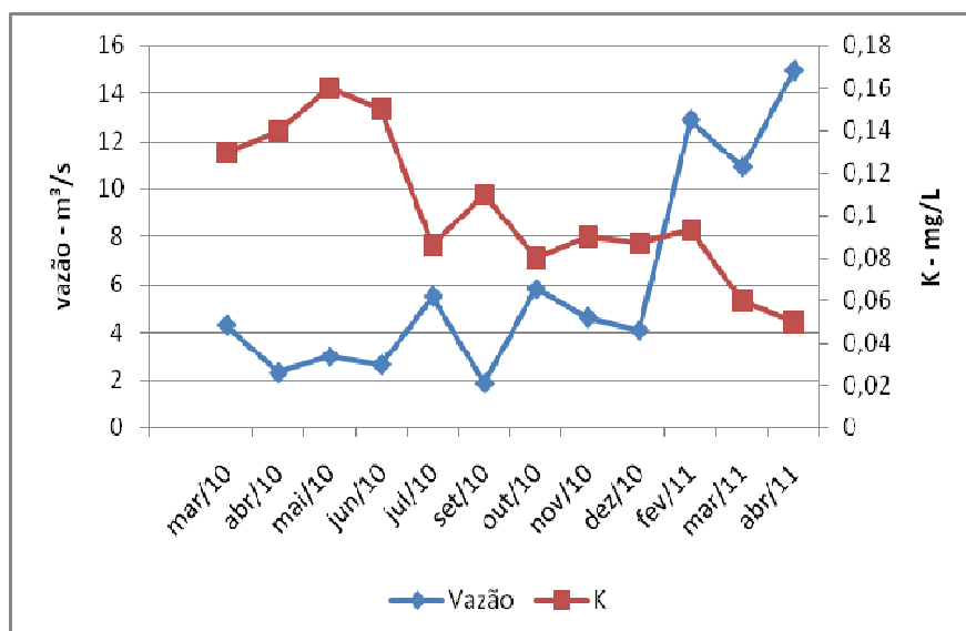
Figura 9 – Relação entre concentração de potássio e a vazão
