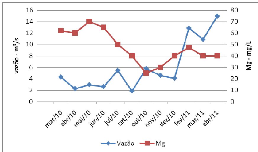
Figura 11 – Relação entre concentração de magnésio e vazão
