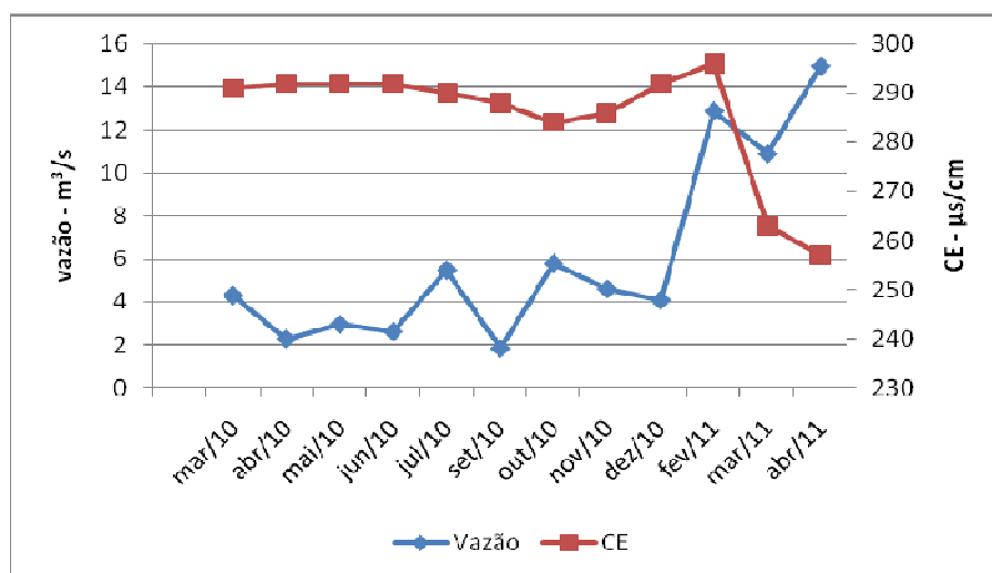
Figura 4 – Relação entre CE e a vazão
