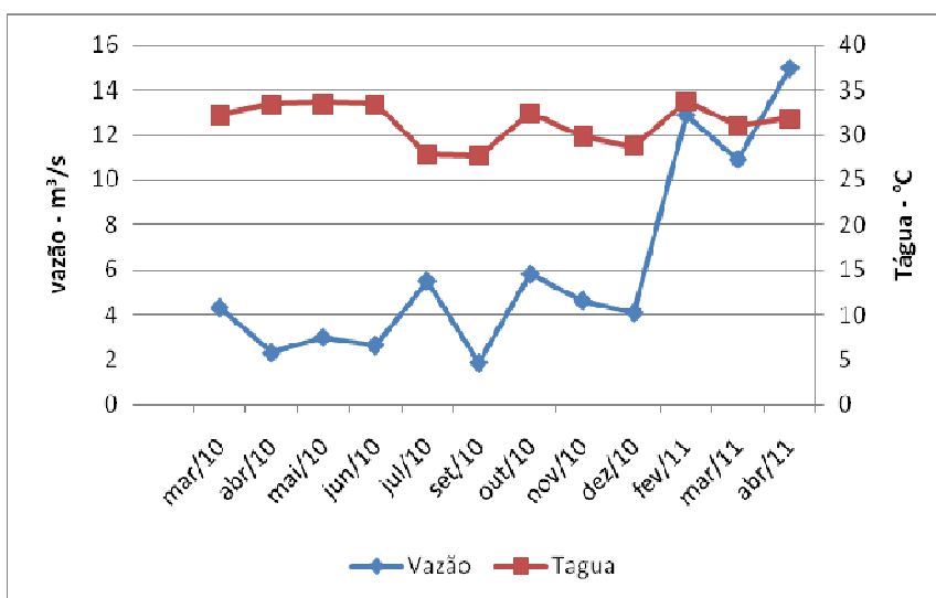
Figura 6 –Relação entre temperatura da água e a vazão
