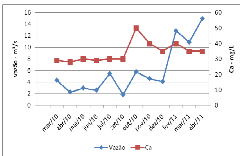
Figura 10 – Relação entre concentração de cálcio e a vazão
