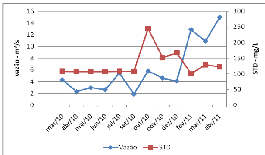
Figura 12 – Relação entre sólidos totais e vazão
