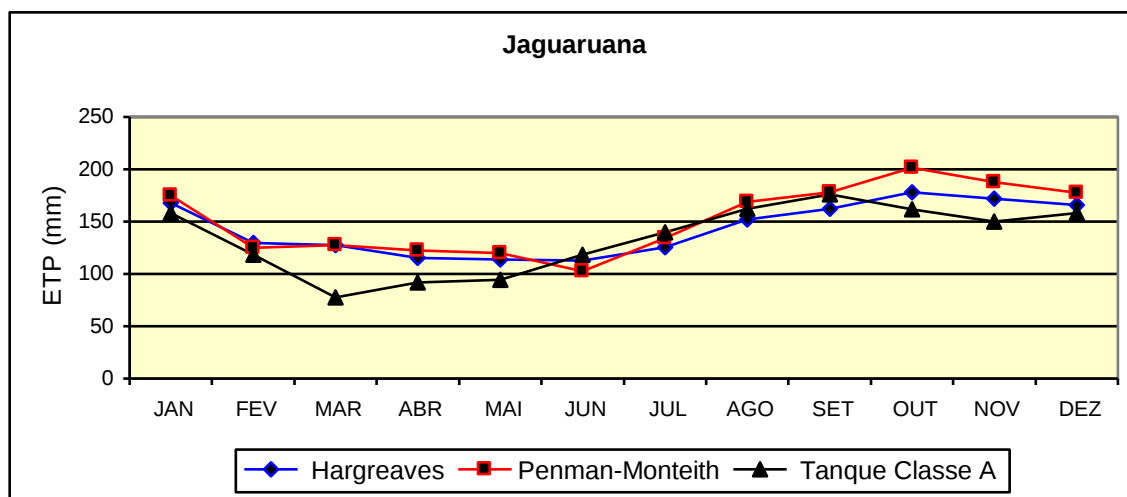
Figura 2 – Evapotranspiração Potencial pelos métodos de Hargreaves, Penman-Monteith e Tanque Classe A em Jaguaruana
