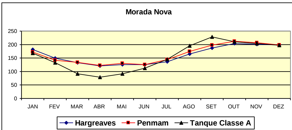
Figura 3 – Evapotranspiração Potencial pelos métodos de Hargreaves, Penman-Monteith e Tanque Classe A em Morada Nova
