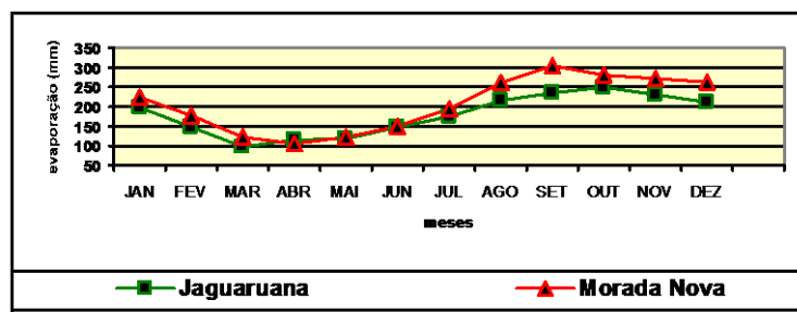
Figura 1 – Evaporação Média nas estações de Jaguaruana e Morada Nova – Tanque Classe A (em mm). Fonte: Ceará (1992)
