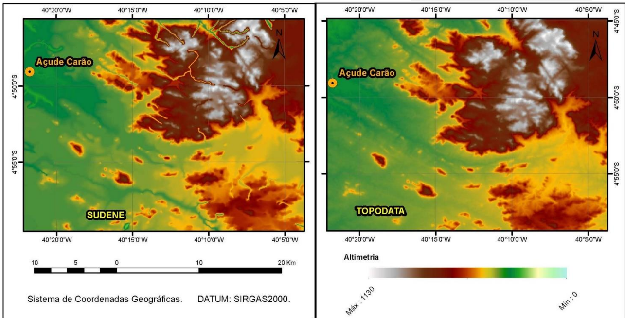
Figura 2 – MDE's gerados na área do açude Carão, com os dados provenientes da SUDENE e do TOPODATA.
