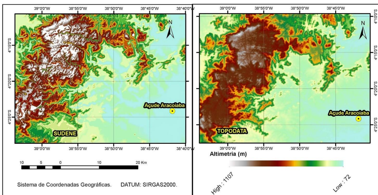
Figura 1 – MDE's gerados na área do Açude Aracoiaba, com os dados provenientes da SUDENE e do TOPODATA.
