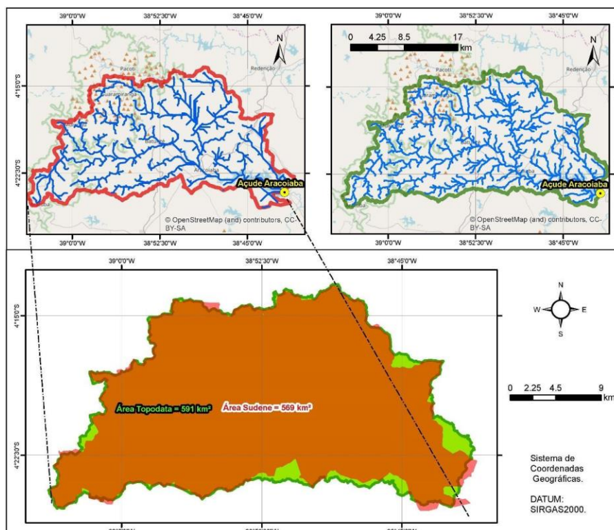
Figura 3 - Bacias hidrográficas do açude Aracoiaba para os dados da SUDENE (esquerda) e TOPODATA (direita).
