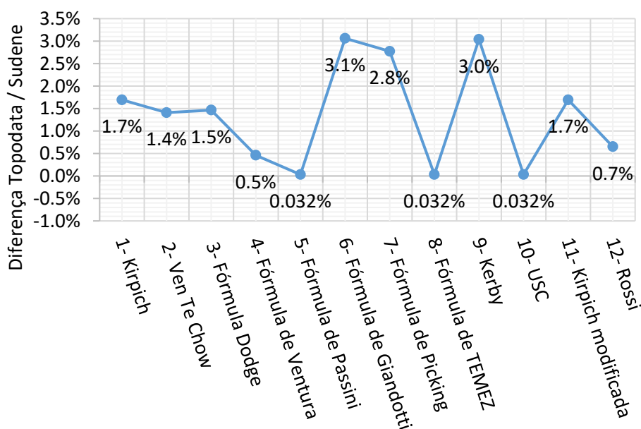
Figura 6 - Diferença entre os tempos de concentração calculados para a bacia do açude Carão.
