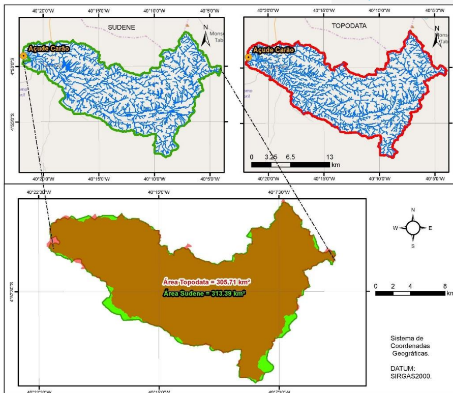
Figura 4 - Bacias hidrográfica do açude Carão para os dados da SUDENE (esquerda) e TOPODATA (direita).
