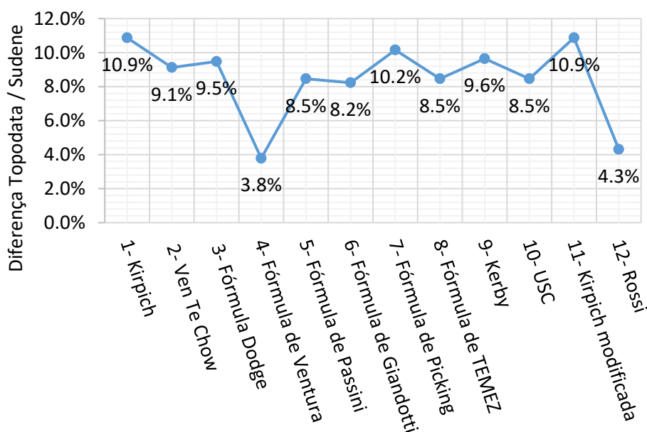
Figura 5 - Diferença entre os tempos de concentração calculados para a bacia do açude Aracoiaba.
