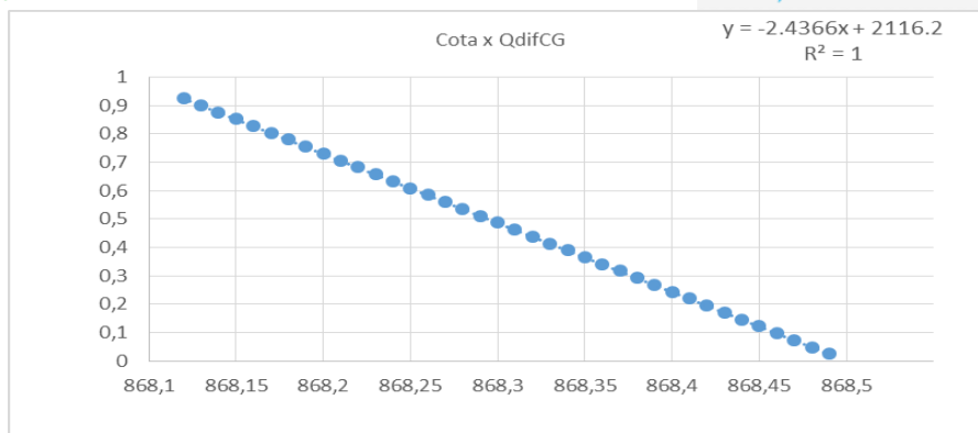
Figura 8: Equação Cota x Volume da represa Cachoeira da Graça.
