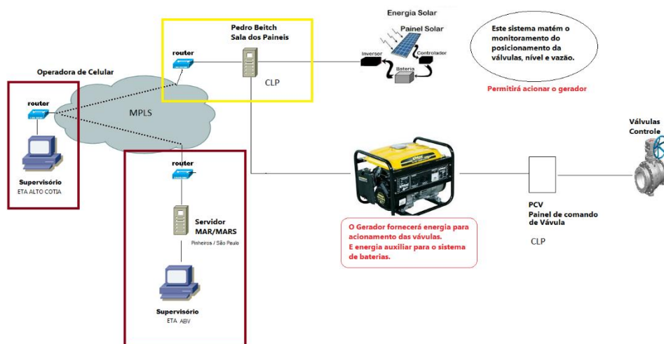
Figura 1 – Croqui do sistema de automação para controle das válvulas de descarga da Barragem Pedro Beicht.
