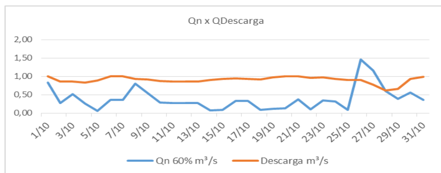
Figura 9: Cálculo da vazão de descarga e a contribuição natural no mês de outubro 2017. Fonte: SSD2 Sabesp.
