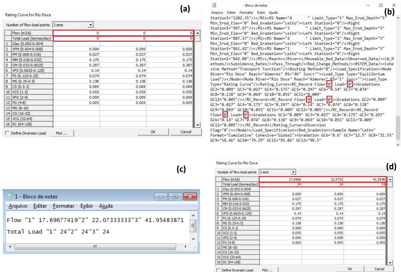
Figura 2 – Sequência de preenchido da curva-chave de sedimentos de forma automática no HEC-RAS: (a) Arquivo do HEC-RAS sem dados de vazões e descargas sólidas totais; (b) Arquivo criado quando se salva um arquivo de curva-chave de sedimentos no HEC-RAS; (c) Curva-chave de sedimentos gerada estocasticamente; (d) Arquivo do HEC-RAS com a curva-chave de sedimentos preenchida de forma automática
